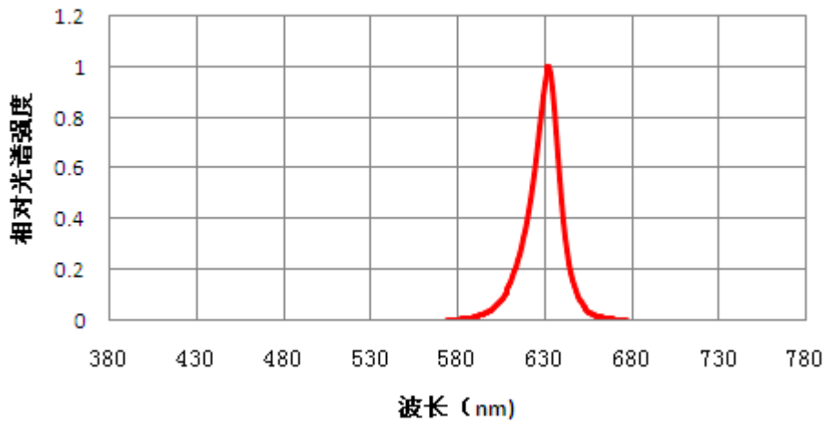
发光角度±5° 相对光谱能量曲线图
