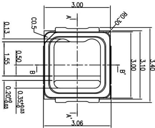
封装尺寸 Package Dimensions
