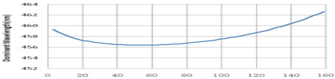
正向电流与主波长曲线
