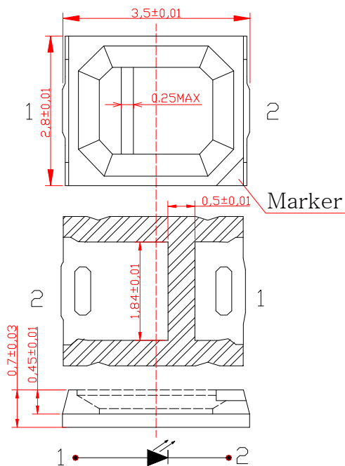
封装尺寸 Package Dimensions
